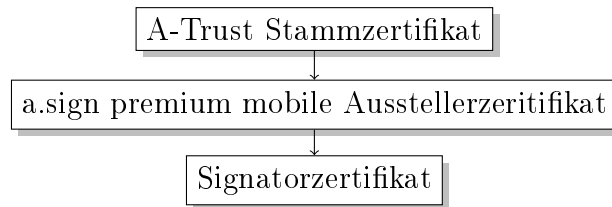
Abbildung 1: Zertifizierungshierarchie
