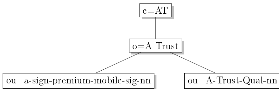
Abbildung 2: A-Trust Verzeichnisbaum
